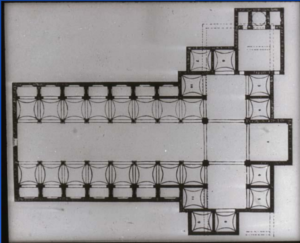
San Lorenzo (Florència) F Brunelleschi
